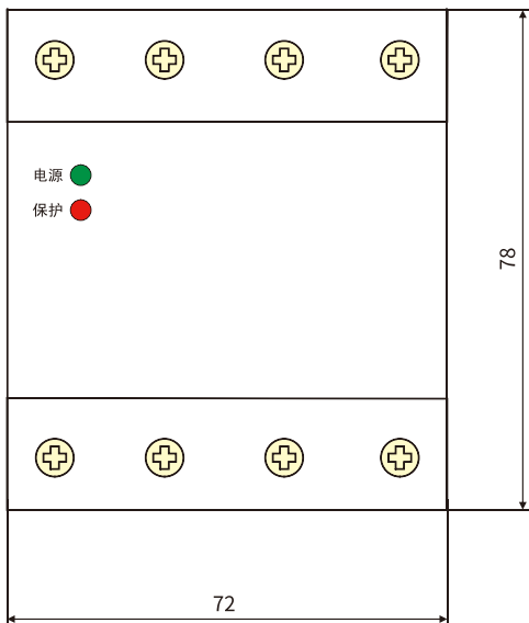
3P+N 外形尺寸
