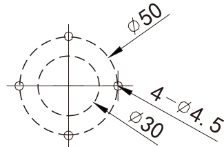
柜外手柄安装开孔尺寸
