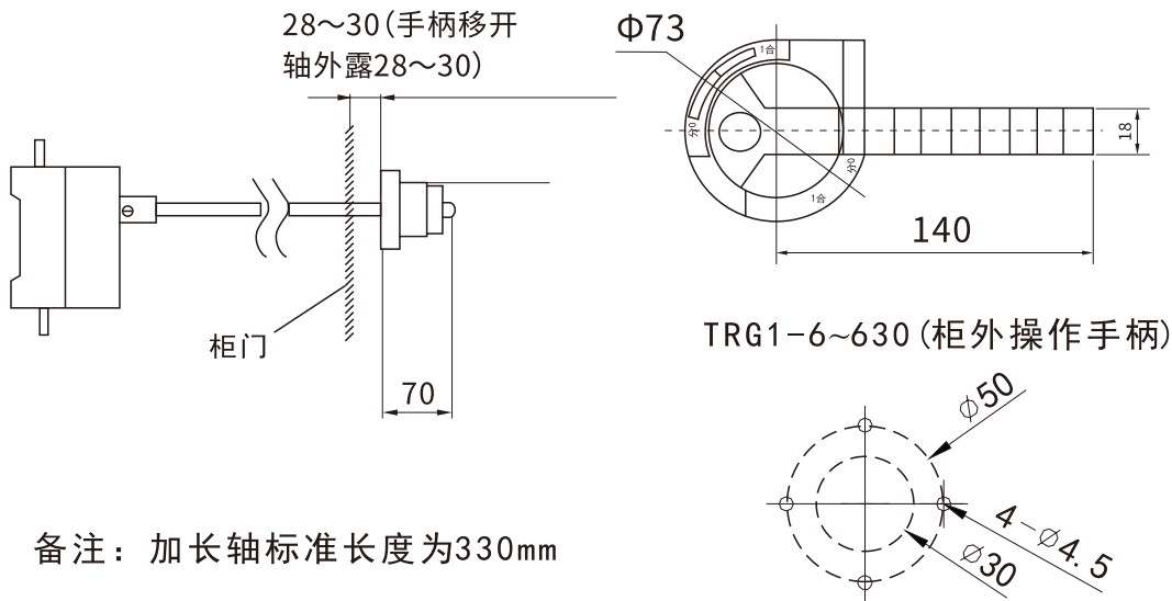
柜外手柄安装开孔尺寸
