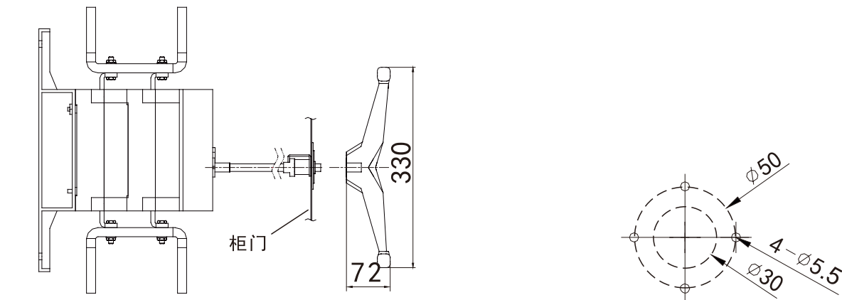
备注：加长轴标准长度为210mm
