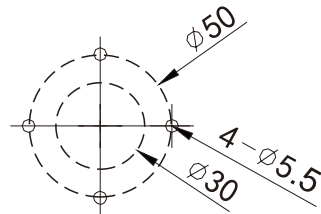
柜外手柄安装开孔尺寸
